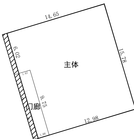
一层平面图
