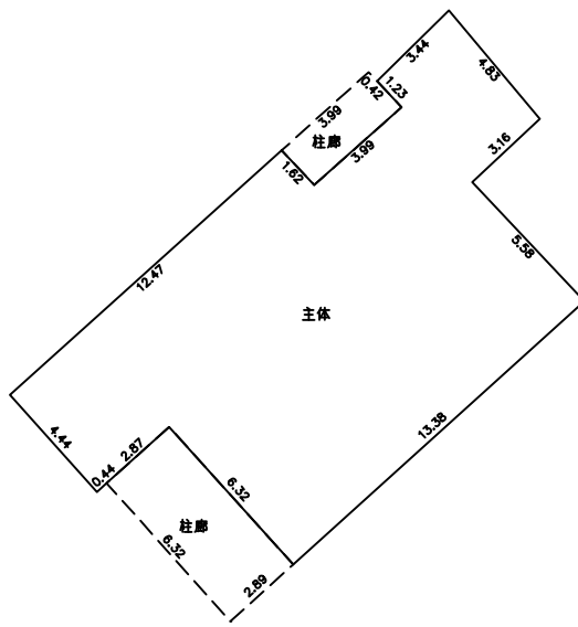
第1层平面图
