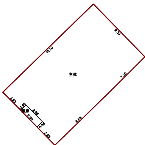
第1层平面图
