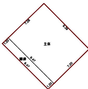
第3层平面图
