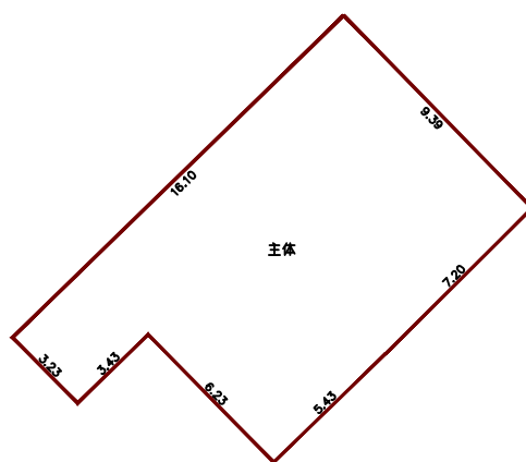
第2层平面图
