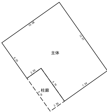
第1层平面图
