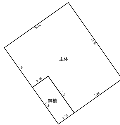
第2层平面图
