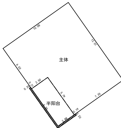
第3层平面图
