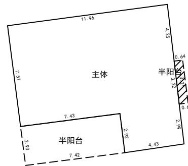
第2层平面图
