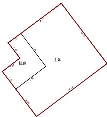
第1层平面图
