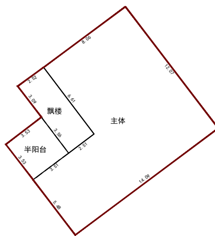
第2层平面图
