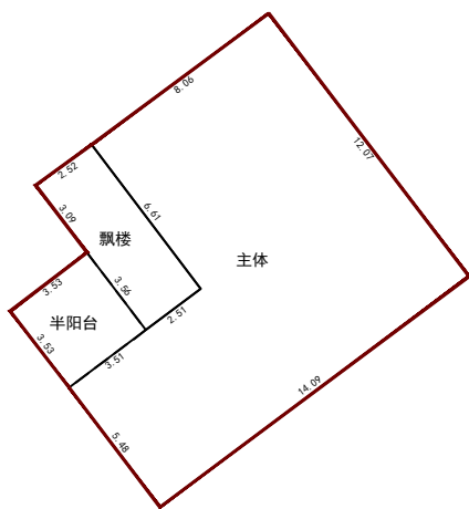
第3层平面图
