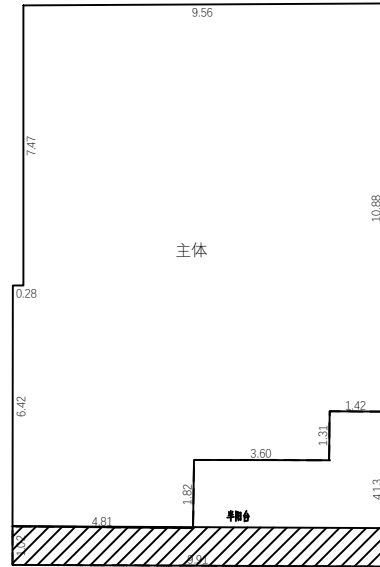
2层平面图
