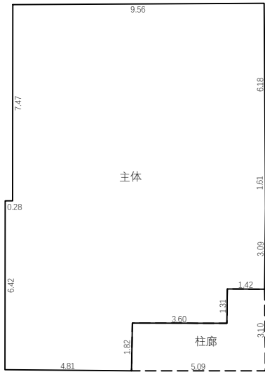
1层平面图
