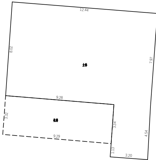
1层平面图
