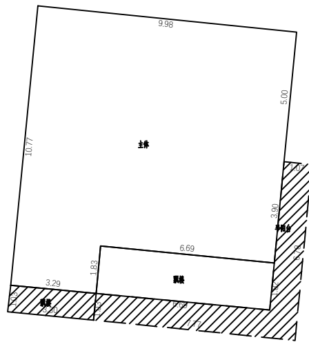
2层平面图
