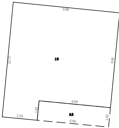
1层平面图
