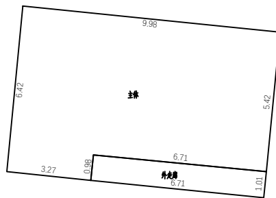
3层平面图
