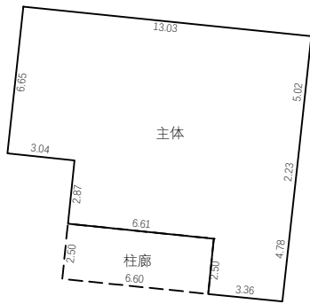
1层平面图
