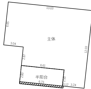
2层平面图
